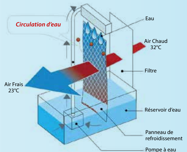
Principe du rafraîchissement d'air par évaporation
